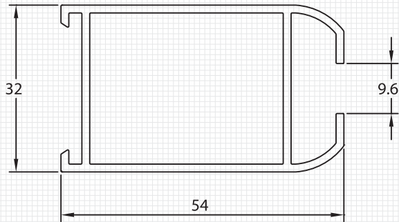
M8811 BASTIDOR MONOLÍTICO Peso : 0.753 Kg./m Espesor : 1.5 mm
